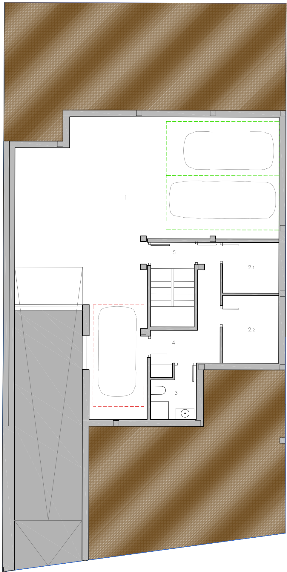
SÓTANO
