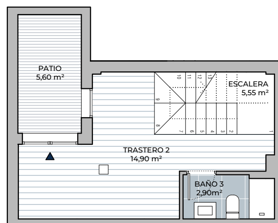
Planta sótano
