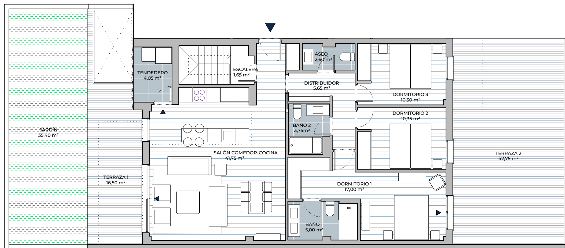
Planta baja
