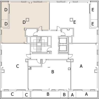
PLANTA 1ª, 2ª, 3ª Y 4ª
